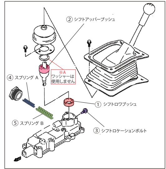
組付け概要
